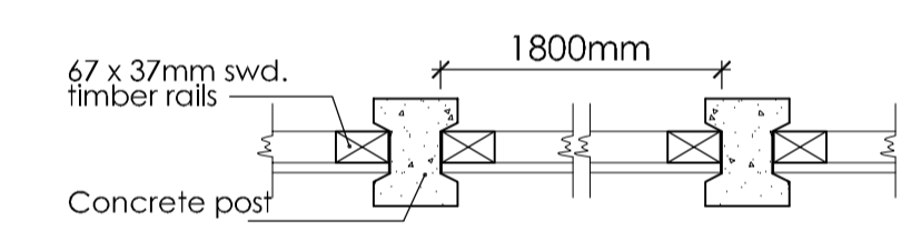
Plan 1:10
