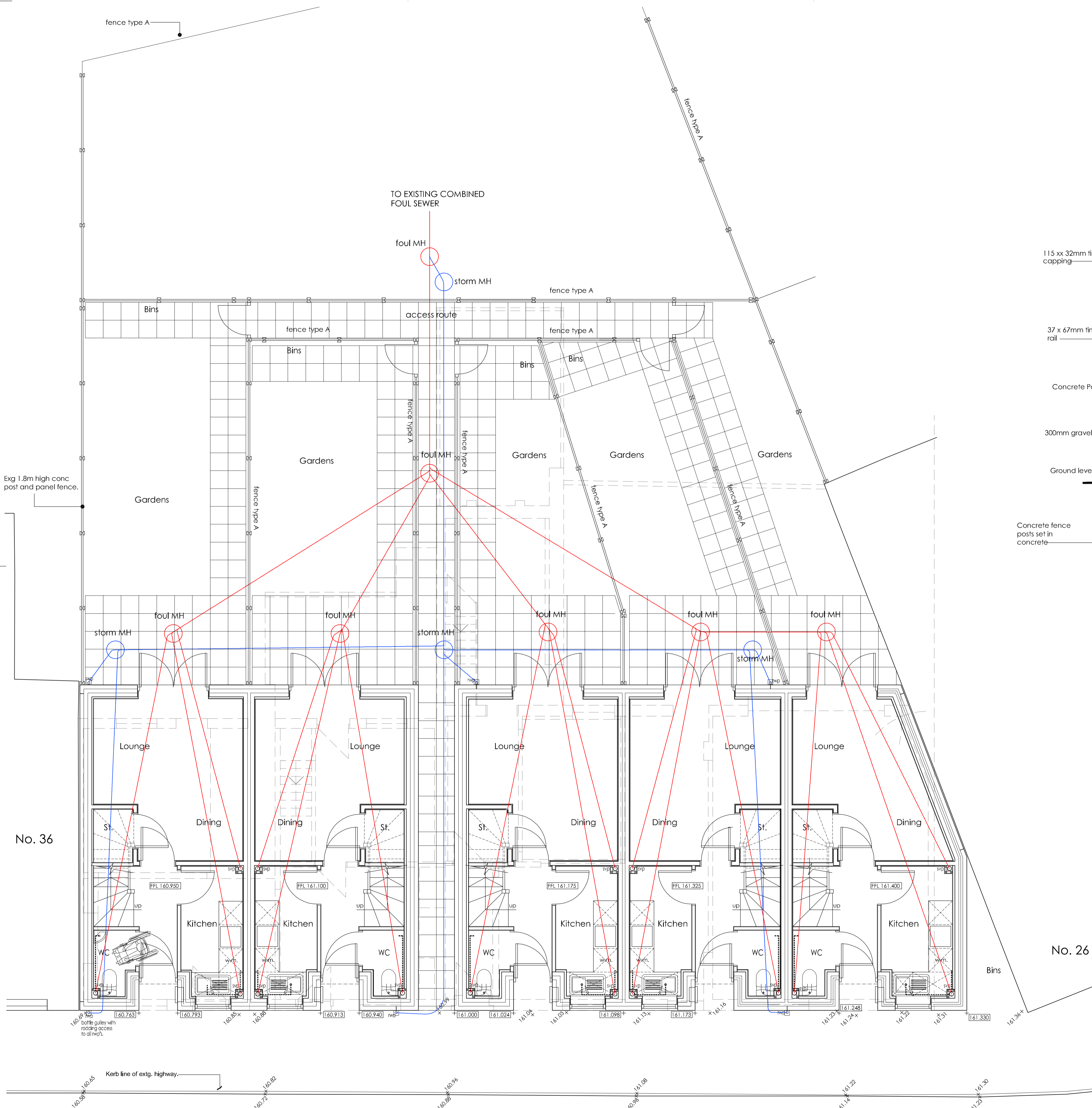
Site plan scale: 1:50
